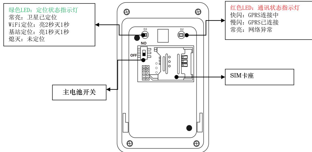
图4.2 主机功能图
